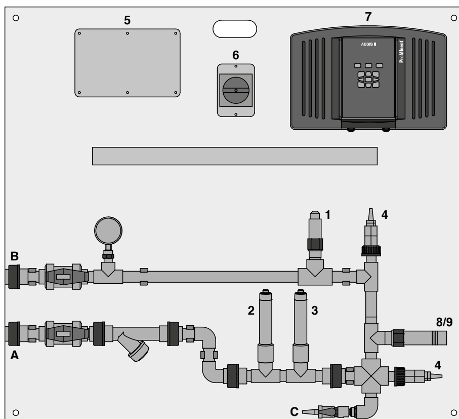
Placa de medición PM AEGIS 2 EU – tipo PM-1, equipamiento de la versión básica, n.º ref. 1093705
