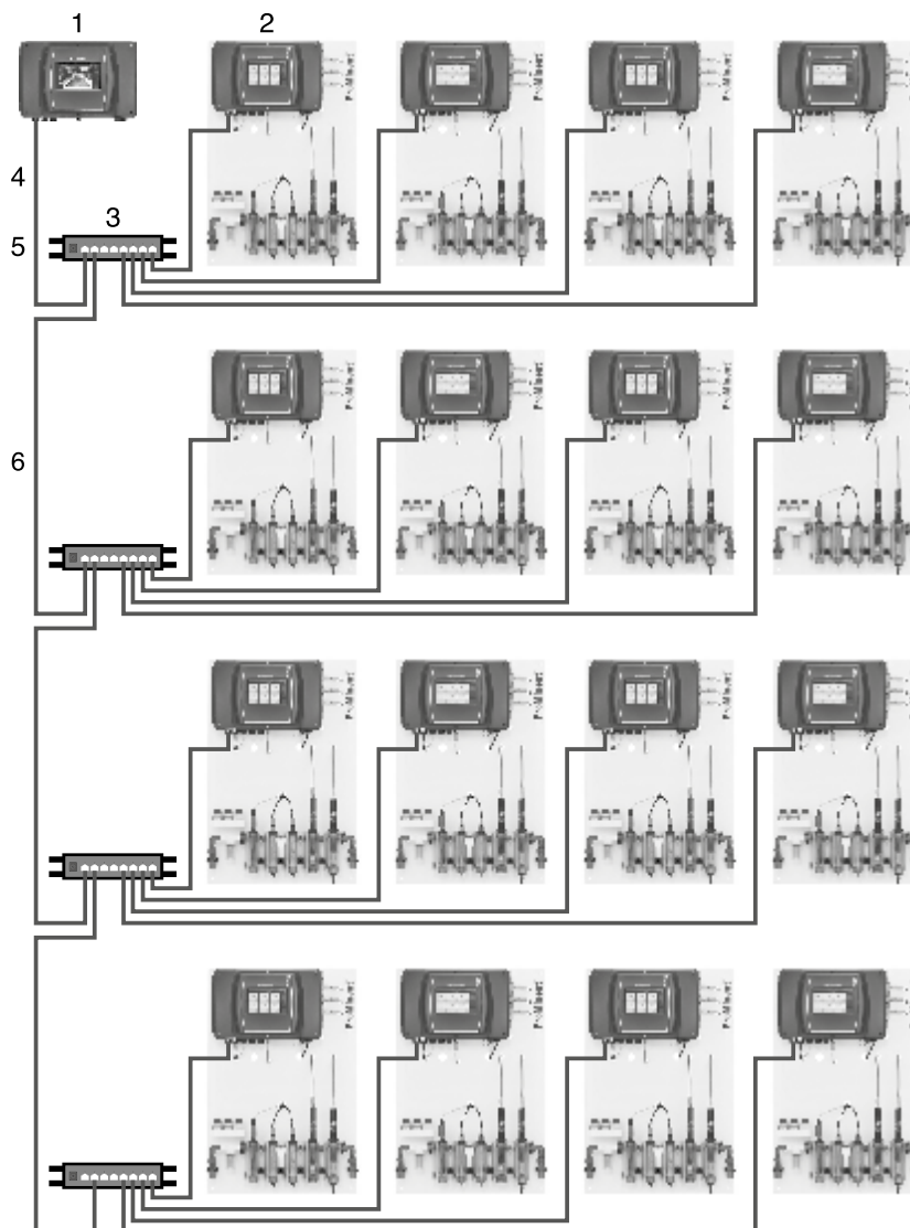
Ejemplo de configuración: Sistema Multipool
