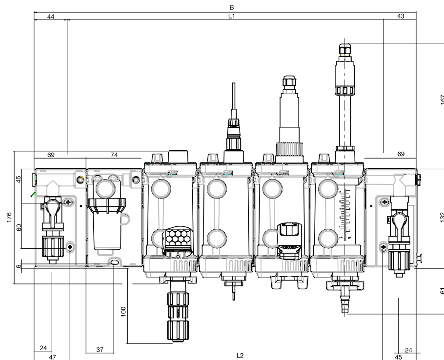
Dimensiones / pesos
